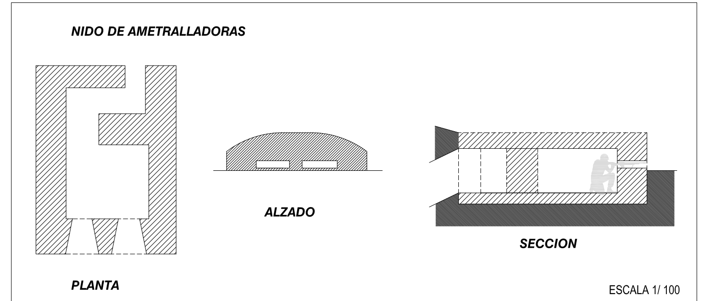
ESQUEMA DE NIDO DE AMETRALLADORAS
